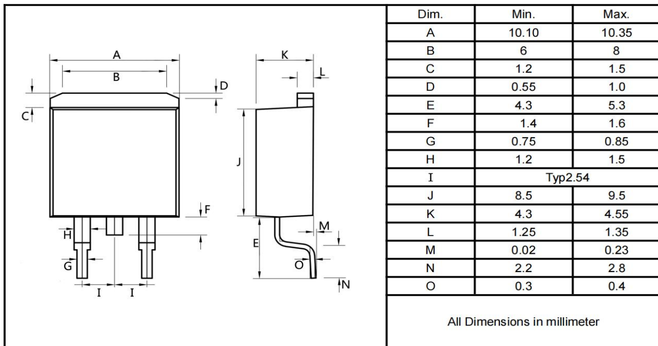
T0-263
